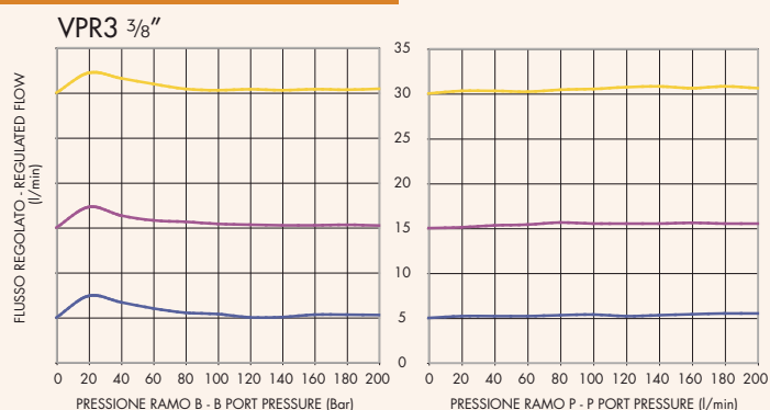
DIAGRAMMA COMPENSAZIONE COMPENSATION CURVE
